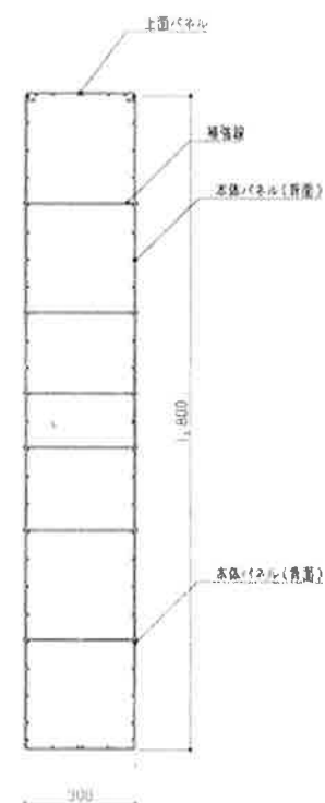
A断面図 S=1:15
