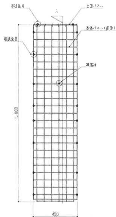
正面図 S=1:15
