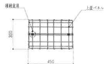
平面図 S=1:15
