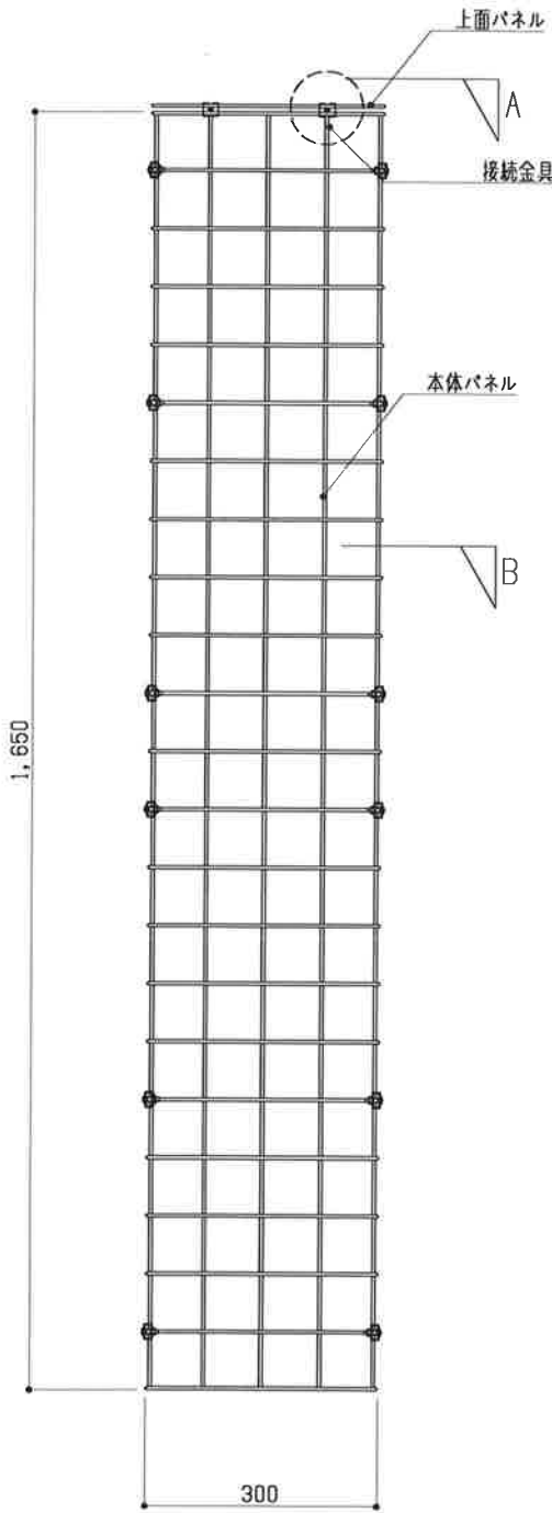
正面図 S = 1 : 10
