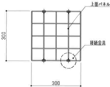
A 断面図 S = 1 : 10
