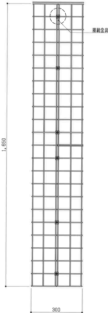
側面図 S = 1 : 10
