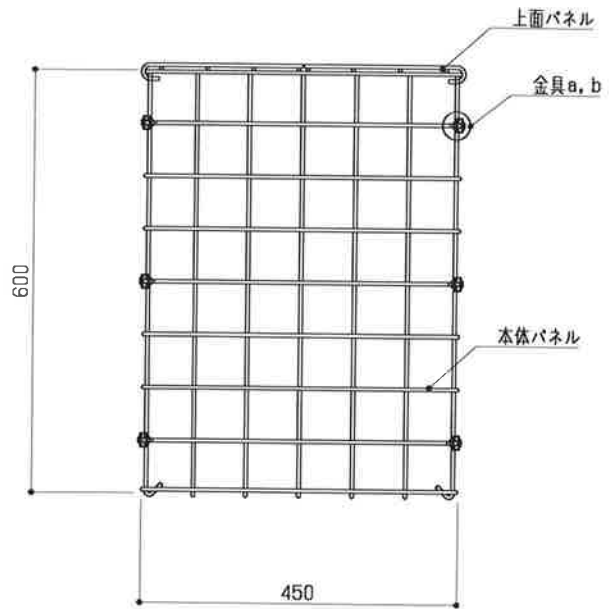
正面図 S = 1 : 10
