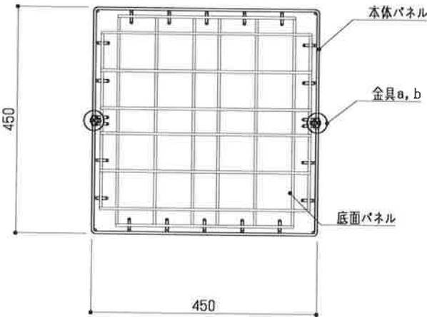
平面図 S = 1 : 10
