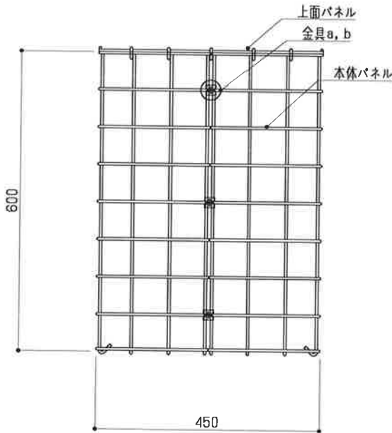
側面図 S = 1 : 10
