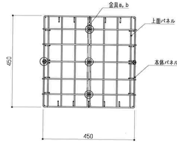
平面図 S = 1 : 10
