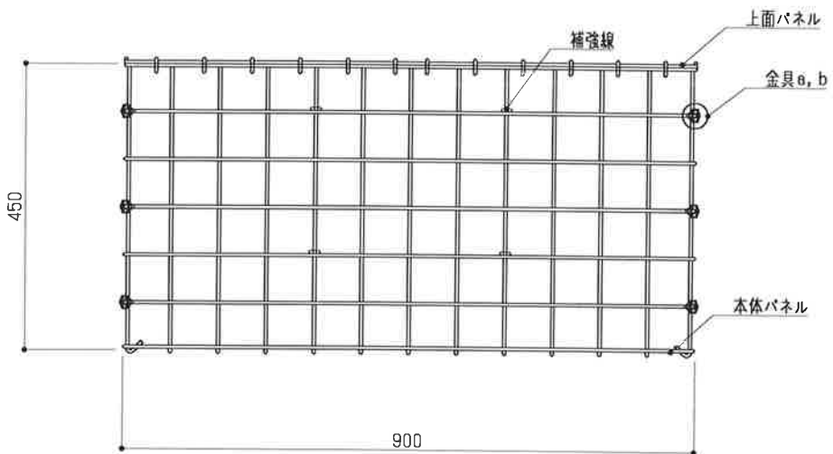
正面図 S=1:10
