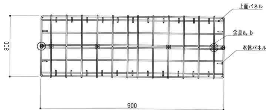
平面図 S=1:10
