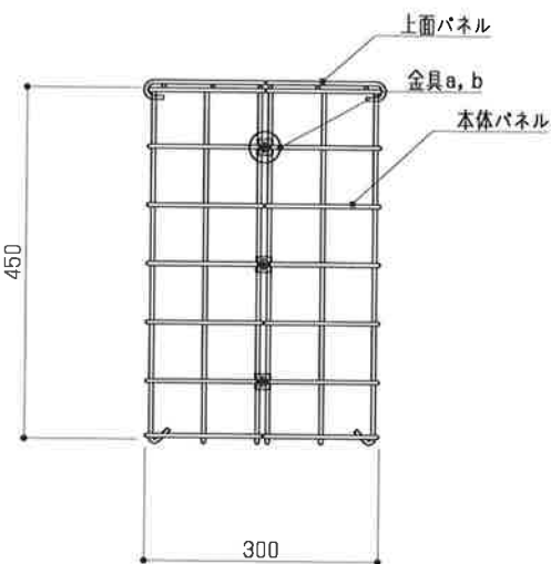
側面図 S=1:10
